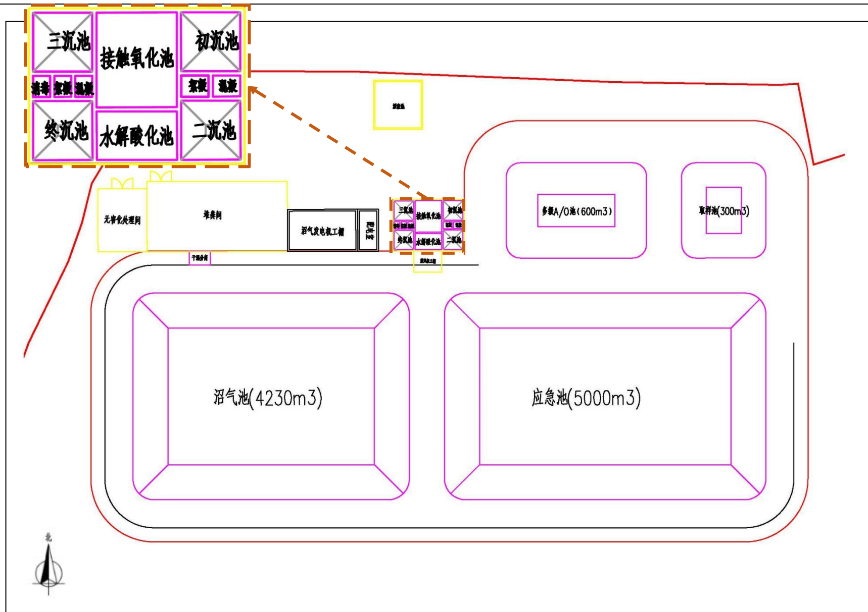
图2.1-3 粪污处理区平面布置图
