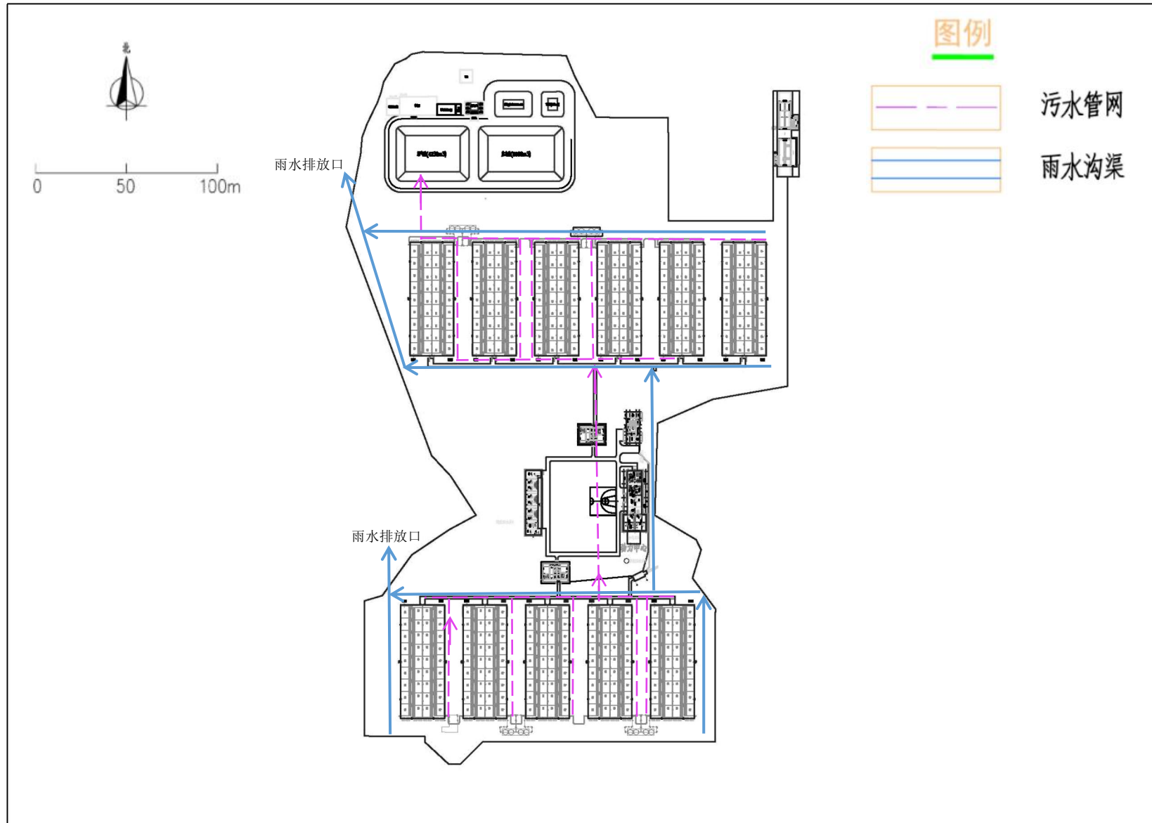
图 2.1-3 厂区雨污管网流向图
