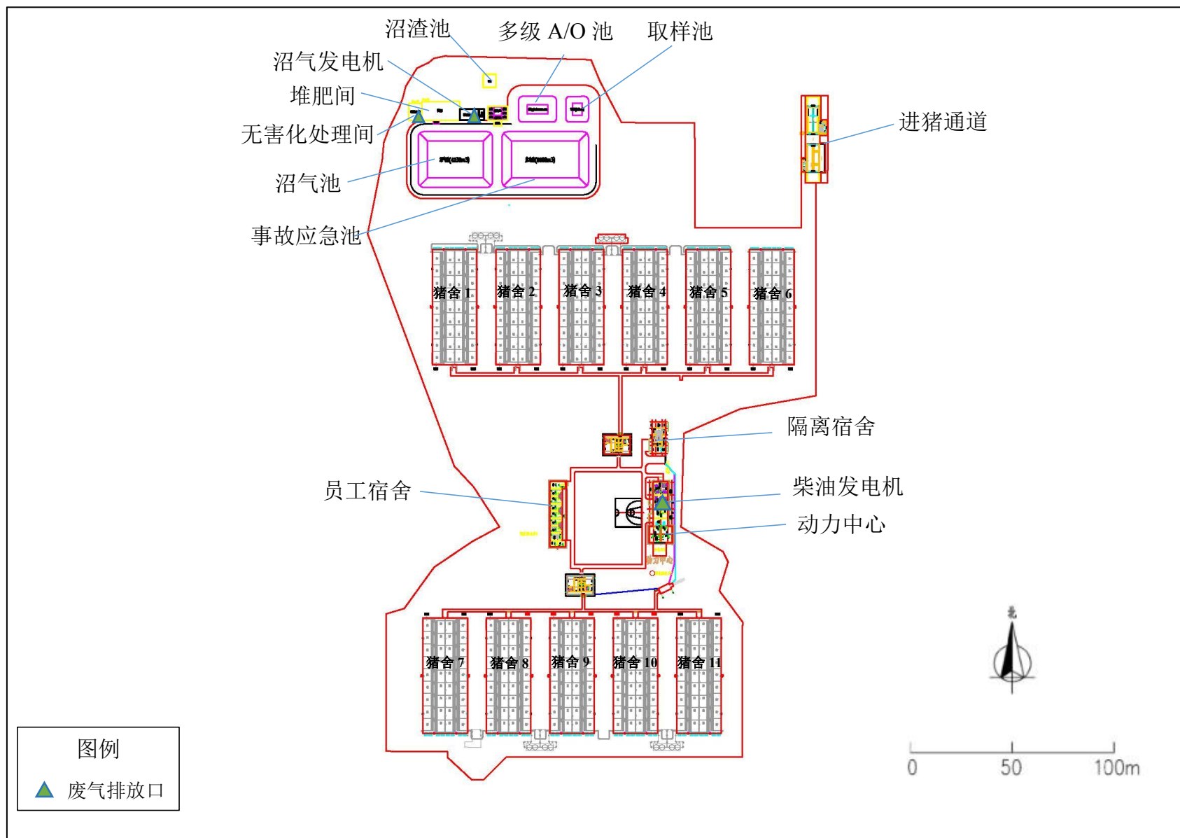
图 2.1-2 项目总平面布置图
