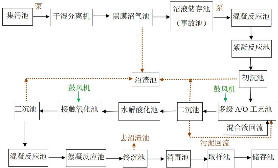
图 6.2-3 废水处理工艺流程示意图
