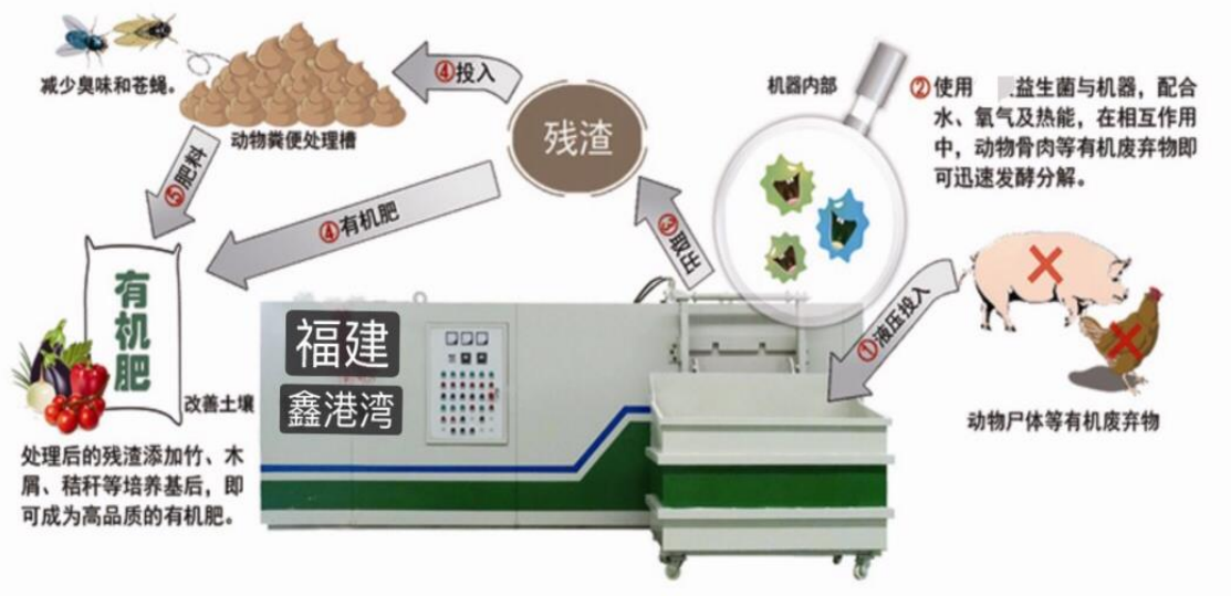
图 2.2-4 病死猪处理工艺流程图
