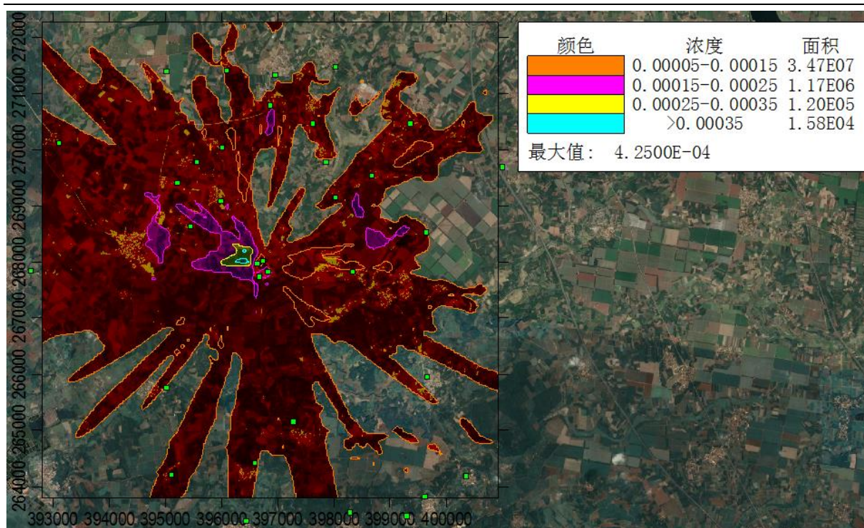
图 5.2-16 PM10 日均浓度预测值分布图
