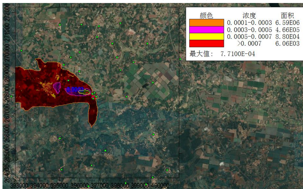
图 5.2-15 NO 2 年均浓度预测值分布图
