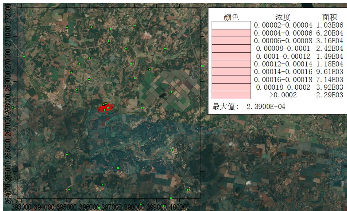
图 5.2-24 非正常工况下 PM 10 日均浓度预测值分布图
