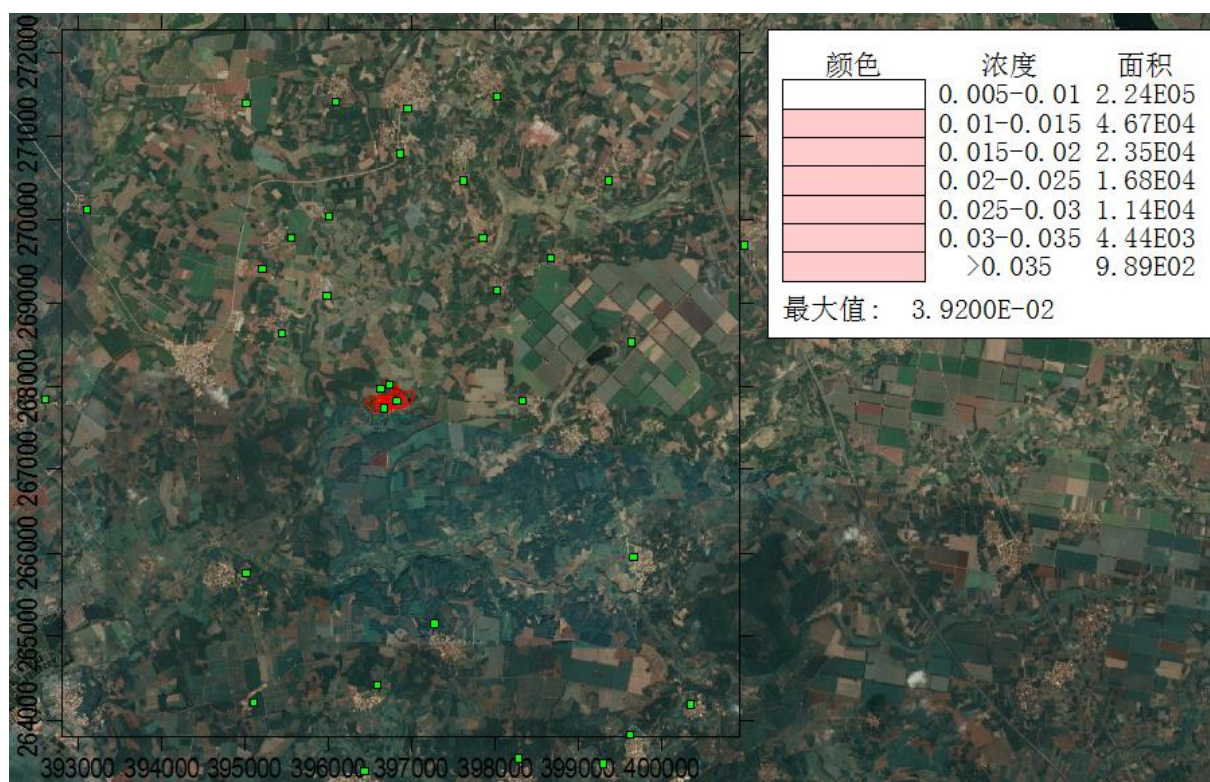
图 5.2-20 非正常工况下 SO 2 日均浓度预测值分布图
