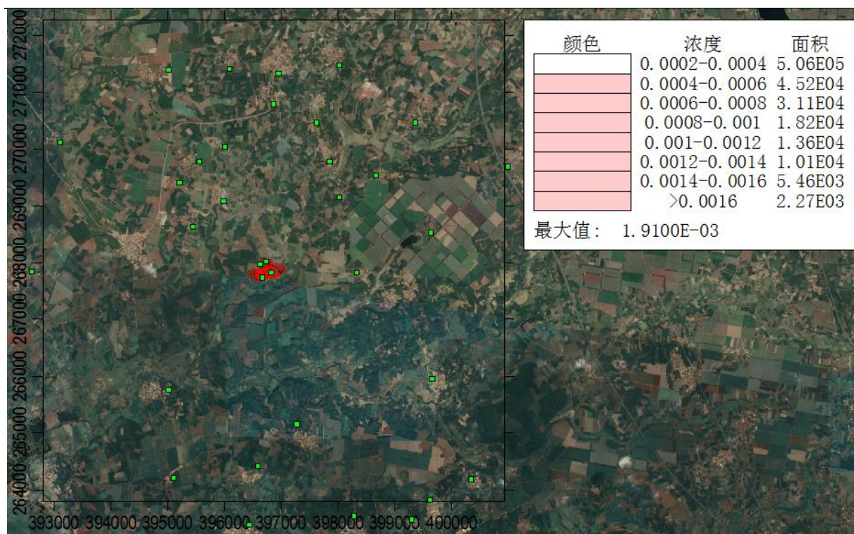
图 5.2-22 非正常工况下 NO 2 日均浓度预测值分布图
