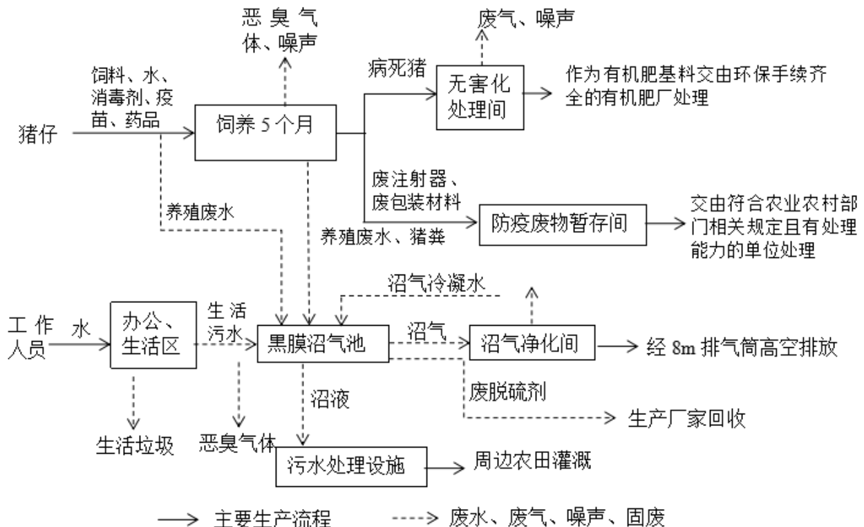
图 2.2-1 生产工艺产排污流程图
