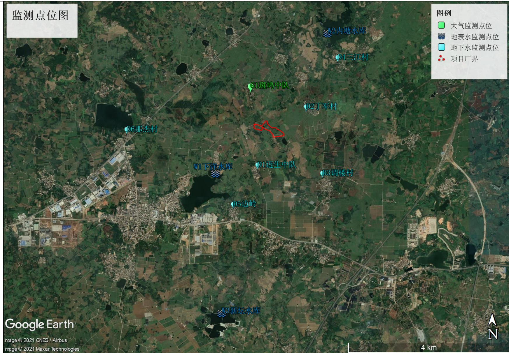
图 4.1-1 项目各要素监测布点图
