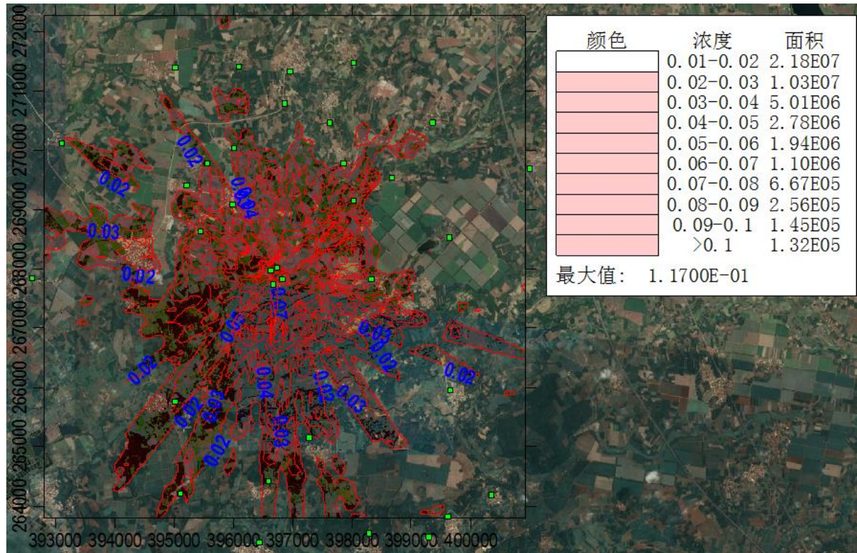
图 5.2-18 非正常工况下 NH 3 小时浓度预测值分布图
