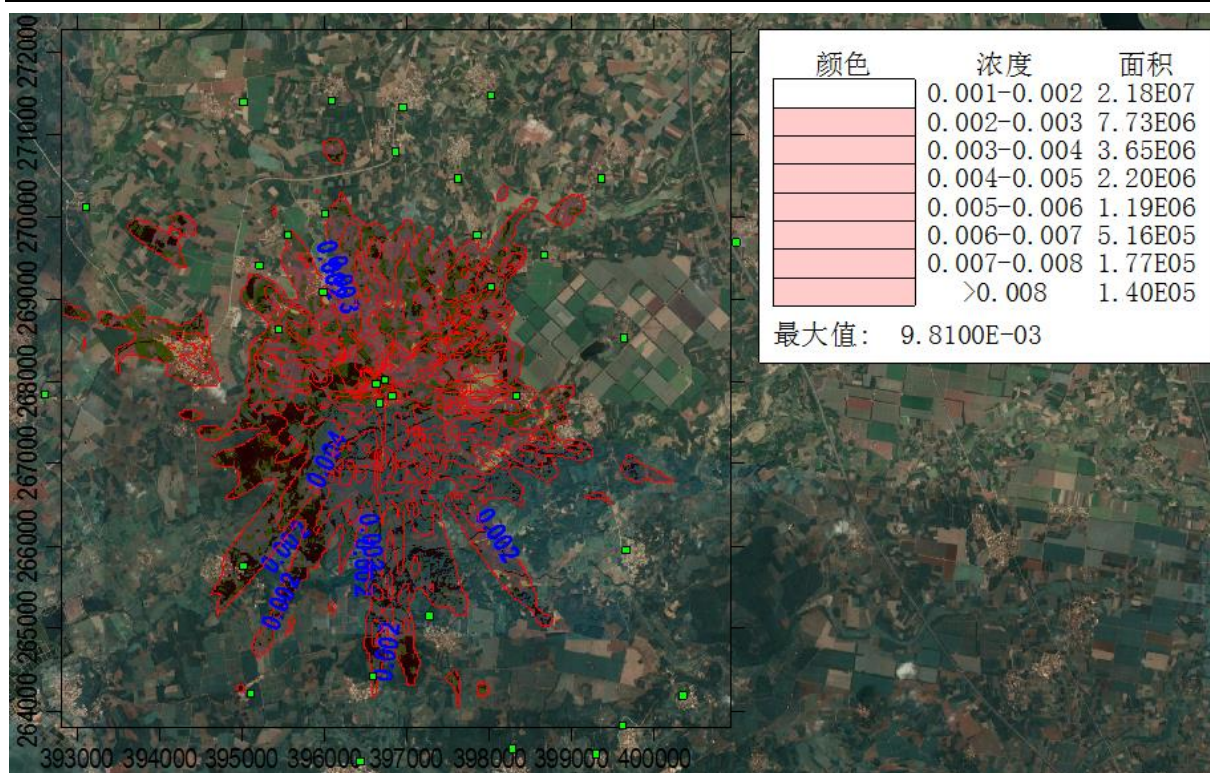
图 5.2-19 非正常工况下 H 2 S 小时浓度预测值分布图
