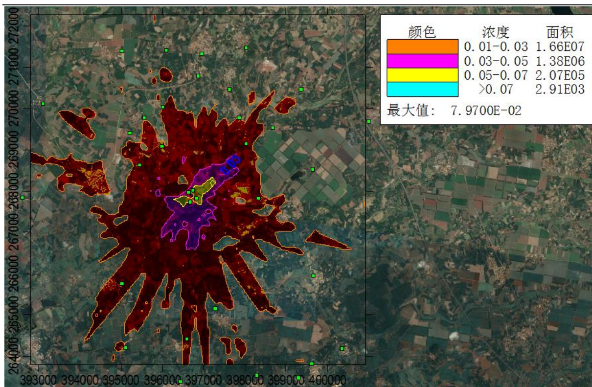
图 5.2-10 NH 3 小时浓度预测值分布图
