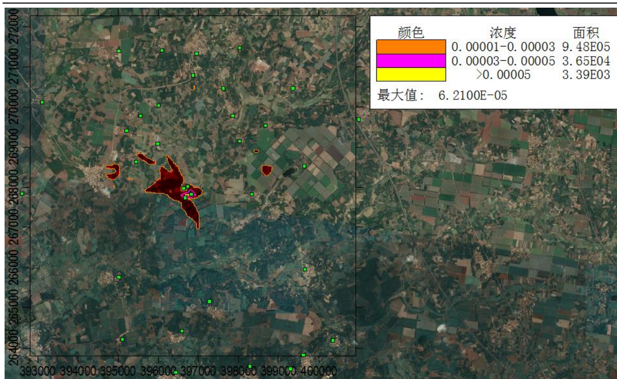
图 5.2-12 SO 2 日均浓度预测值分布图
