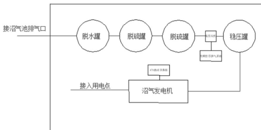
图 2.2-4 沼气发电系统流程图
