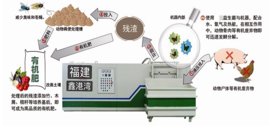
图 2.2-5 病死猪处理工艺流程图
