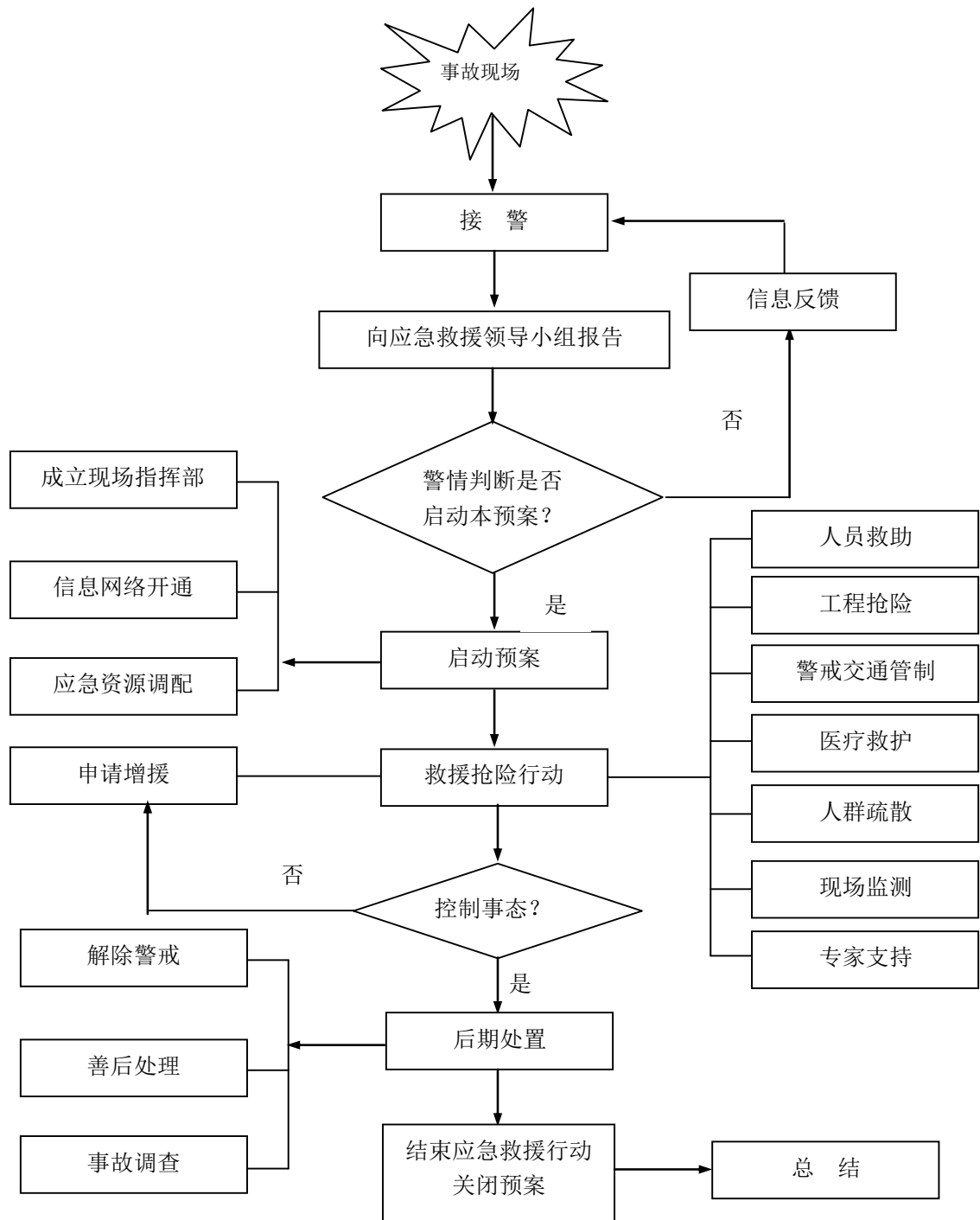
图 5.2-3 报警与响应流程图
