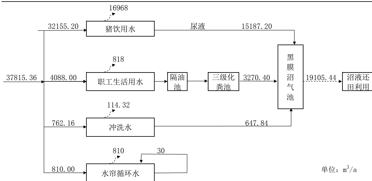
图 2.2-6 项目水平衡图
